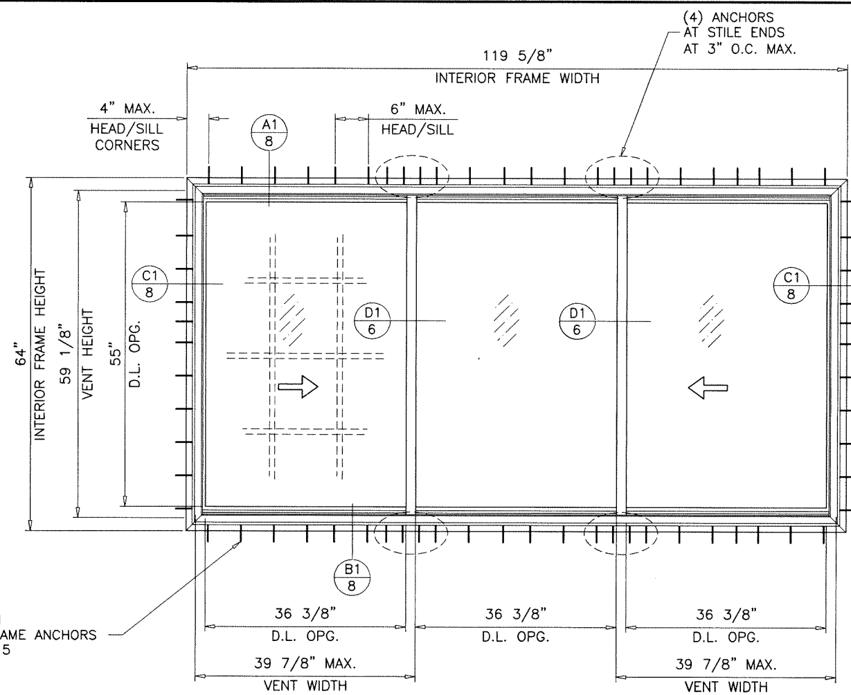
FLUSH FRAMES
